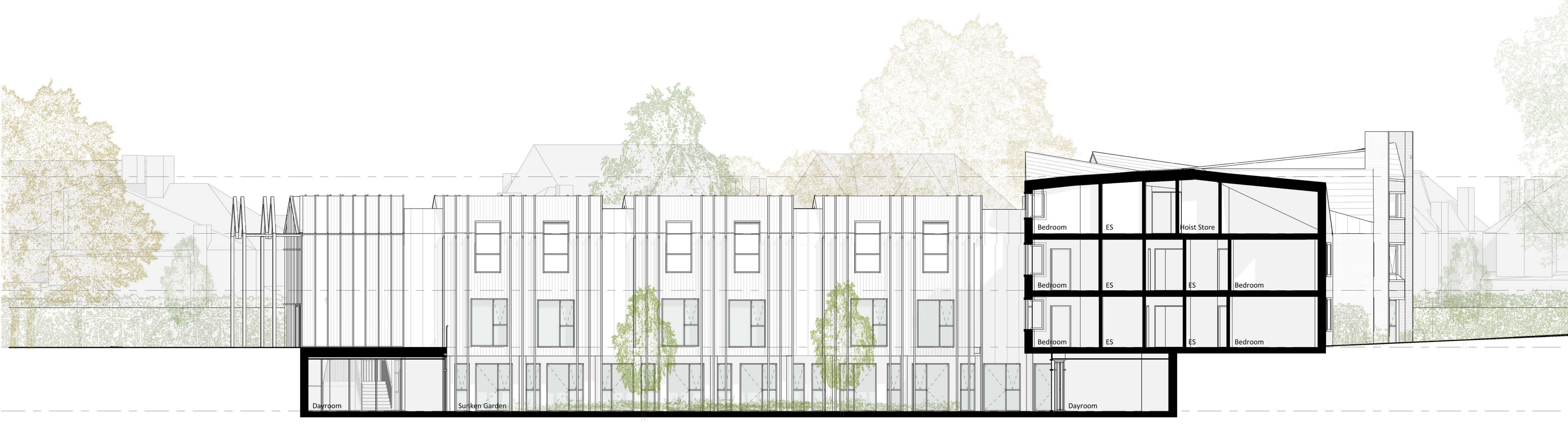
Section A 1 : 100
