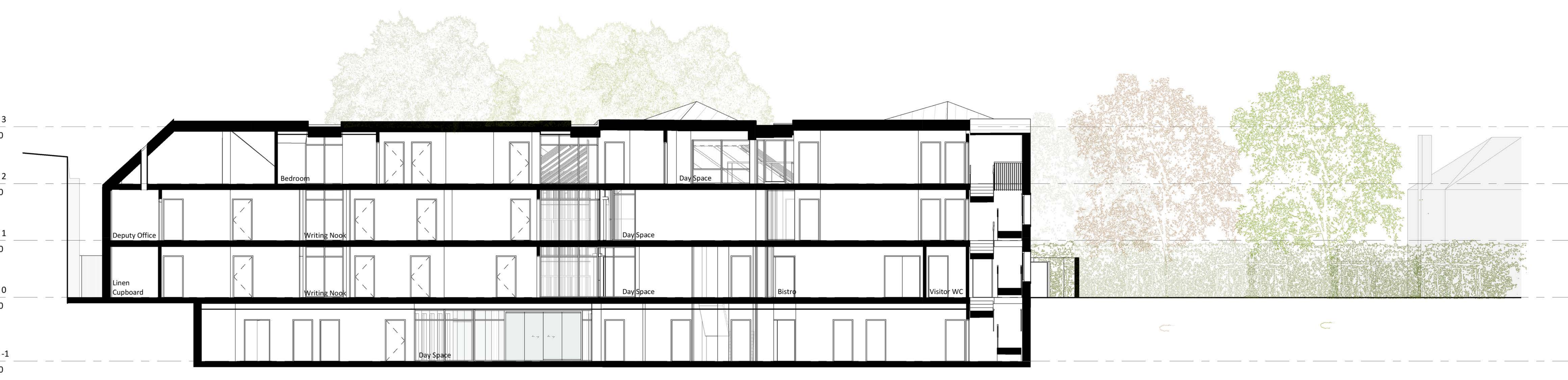
Section D 1 : 100
